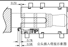
公头插入母座示意图
