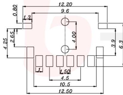
P.C.B LAND DIMENSION
