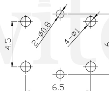
PCB. 焊接尺寸图
