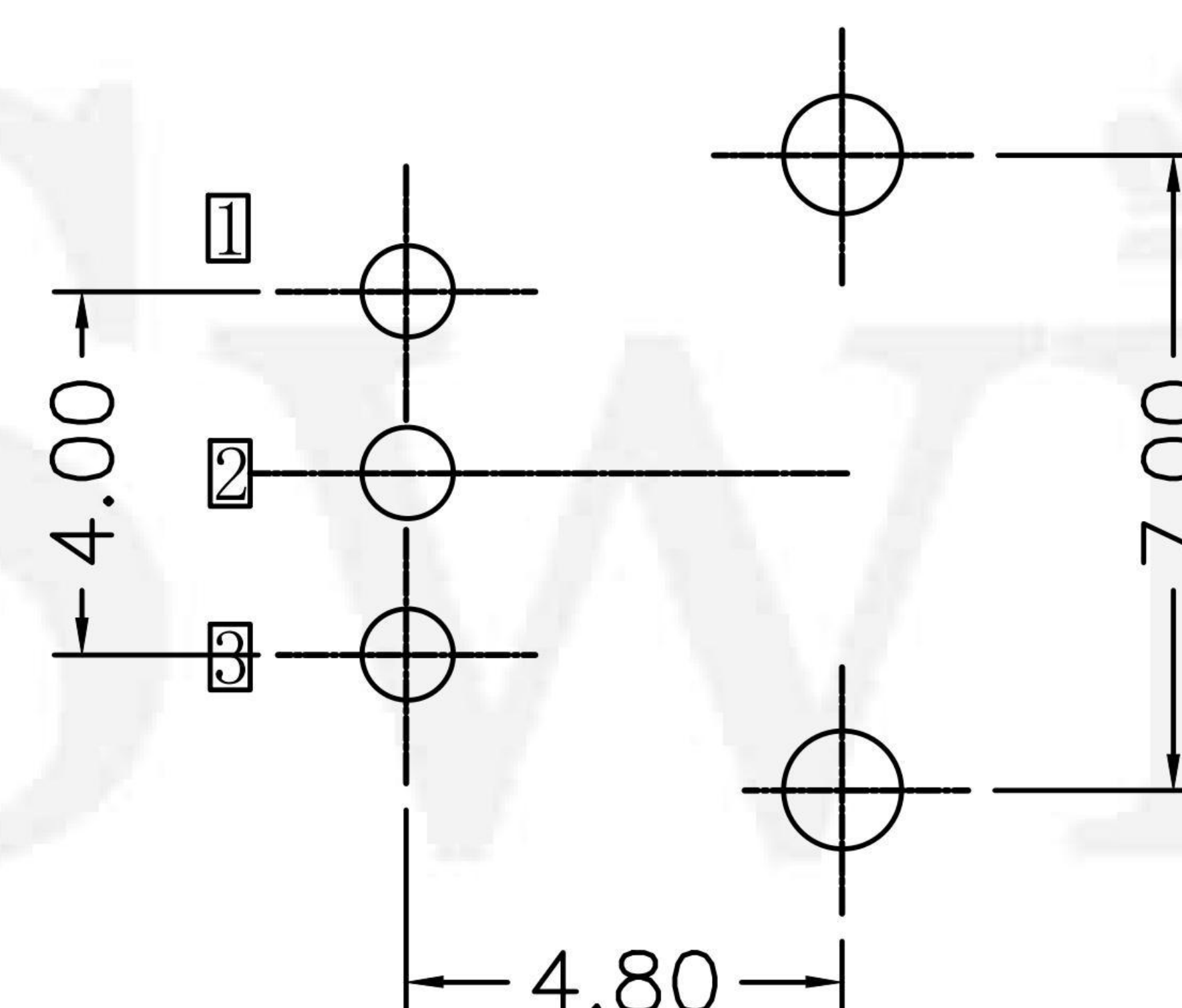
P.C.B LAYOUT
