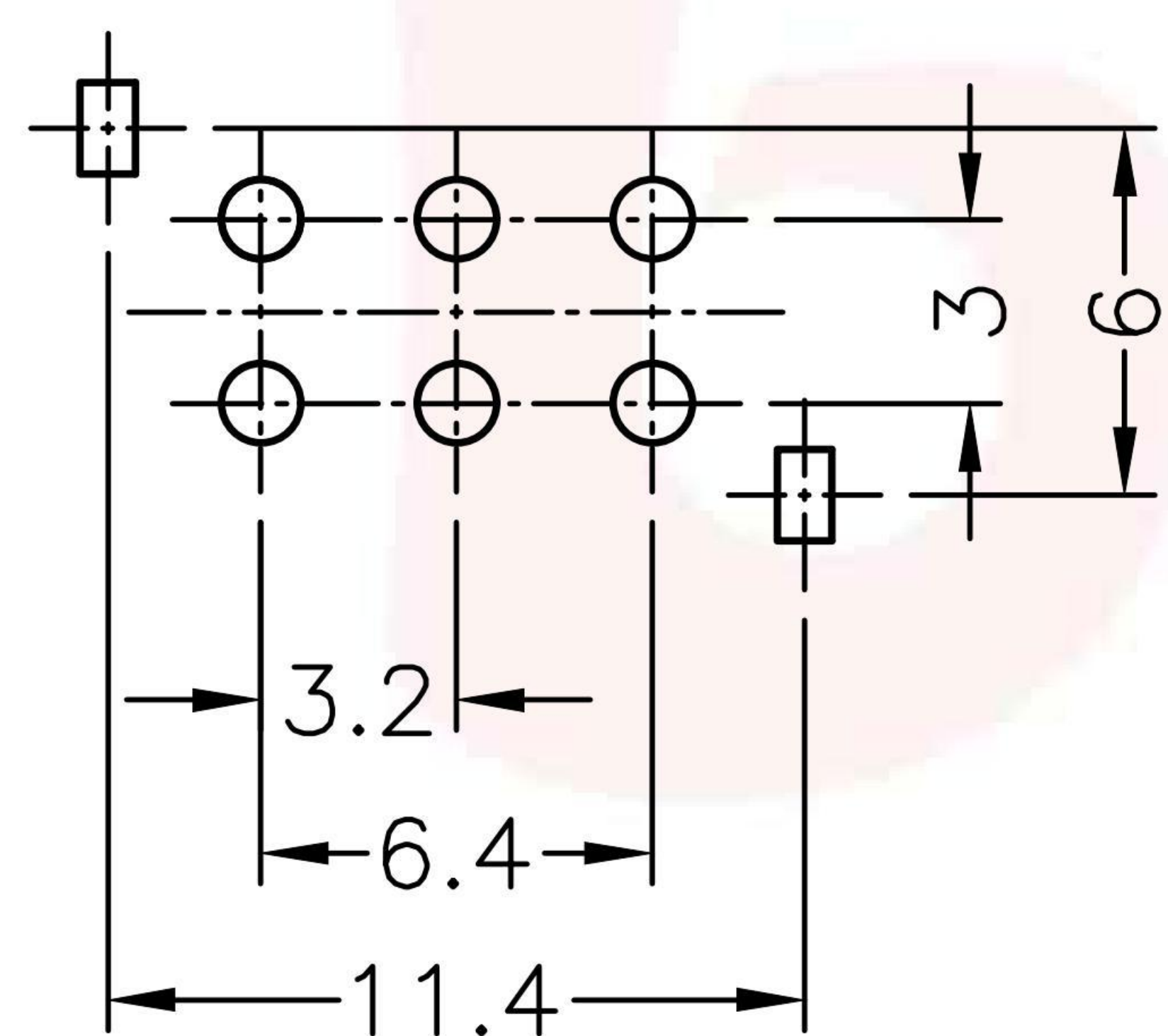
P.C.B LATOUT BOTTOM VIEW
