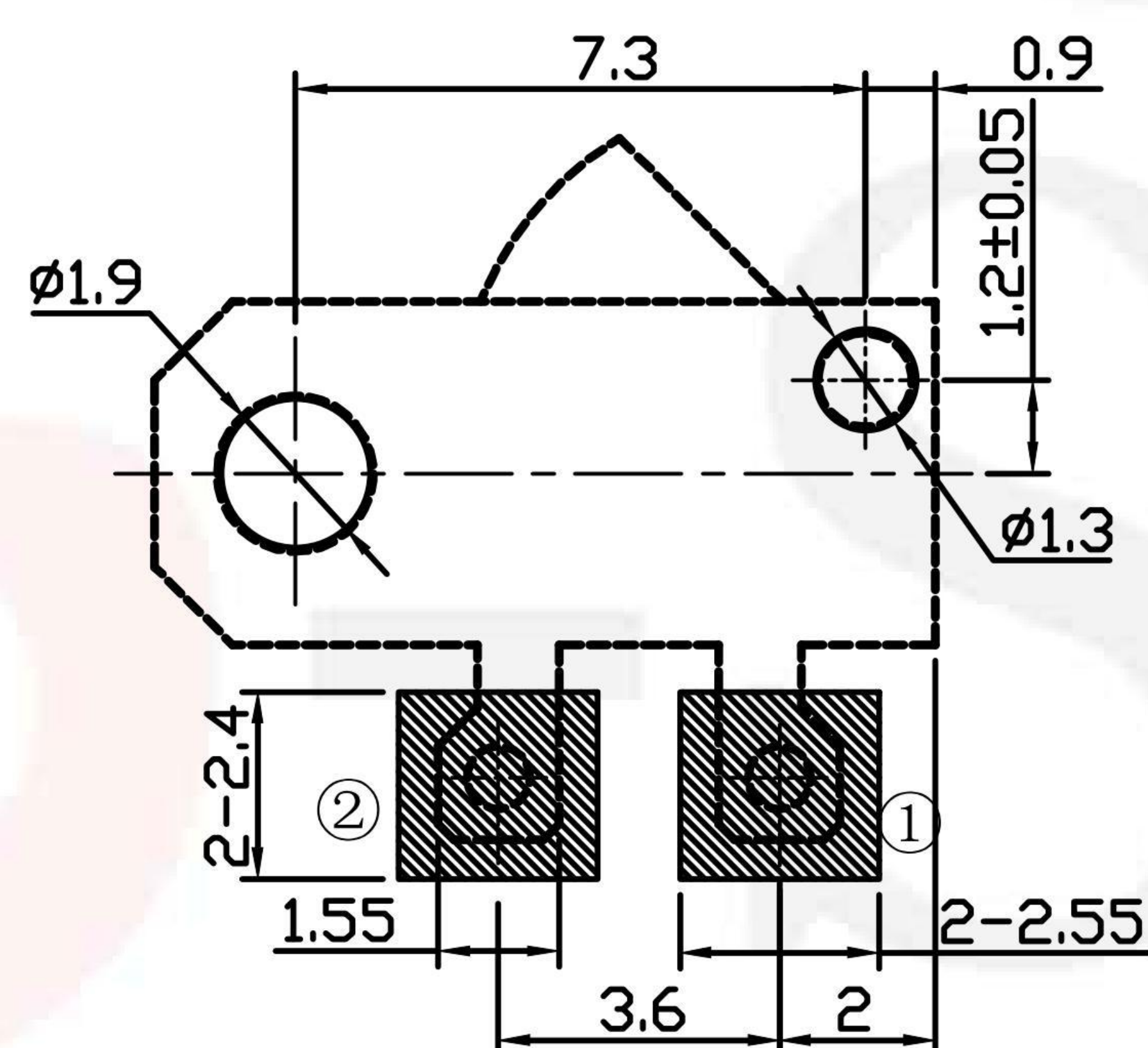
安装位置图
