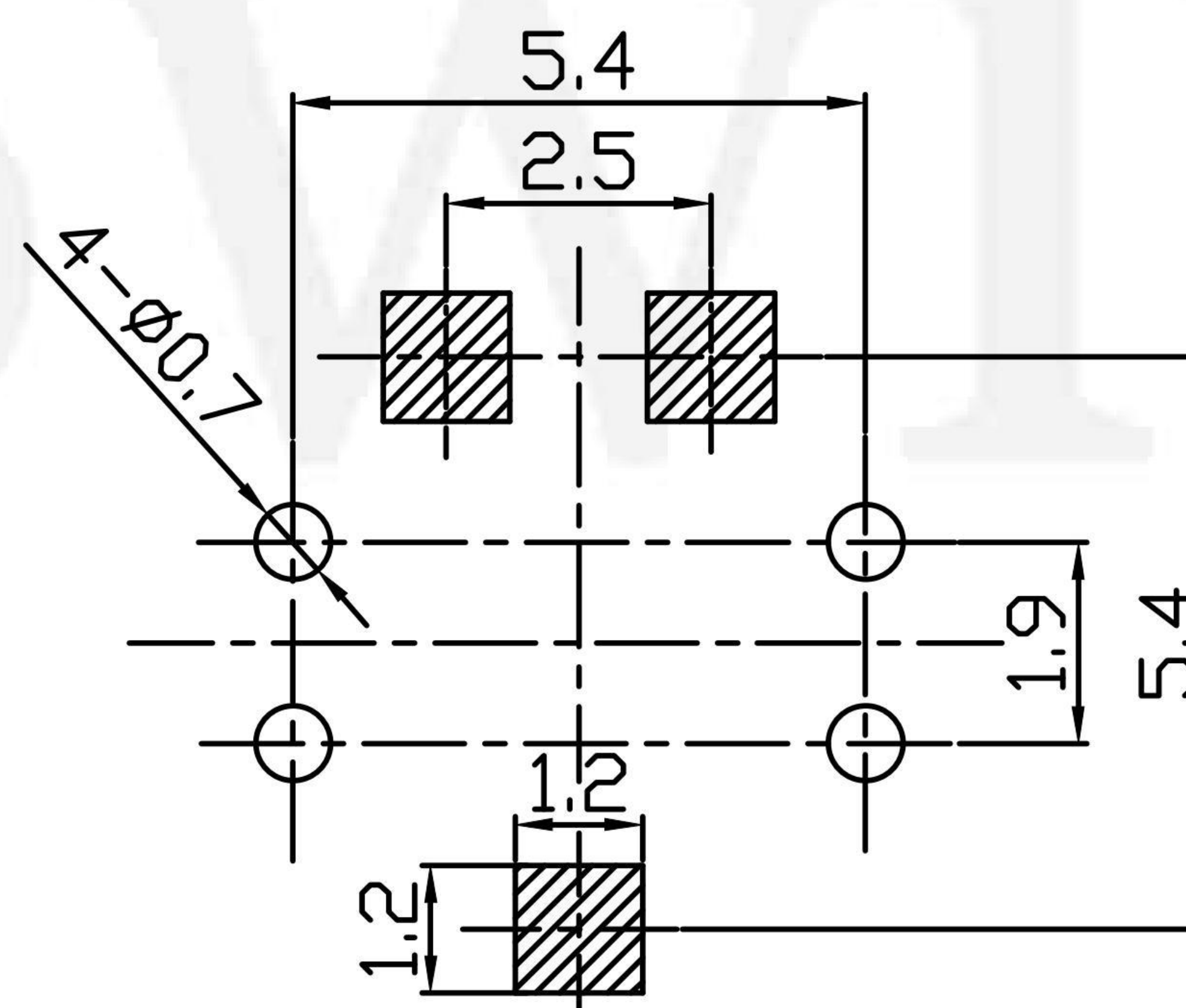
安装尺寸图
