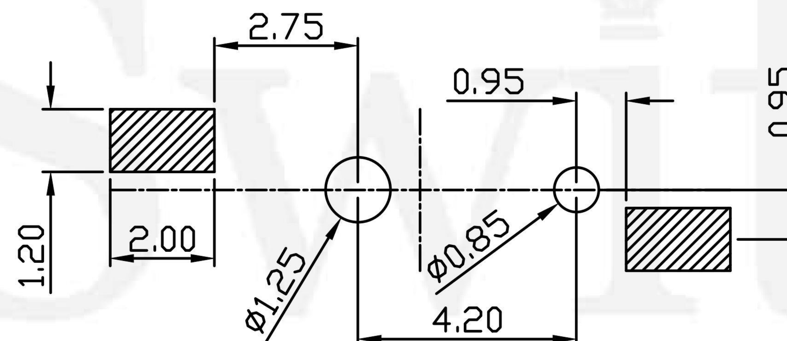
PCB. 焊接尺寸图
