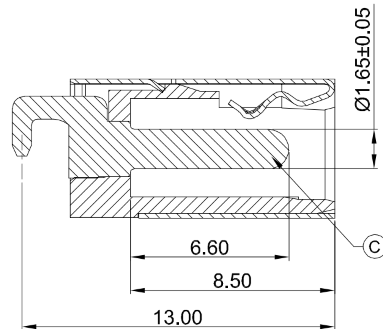
SECTION A-A
