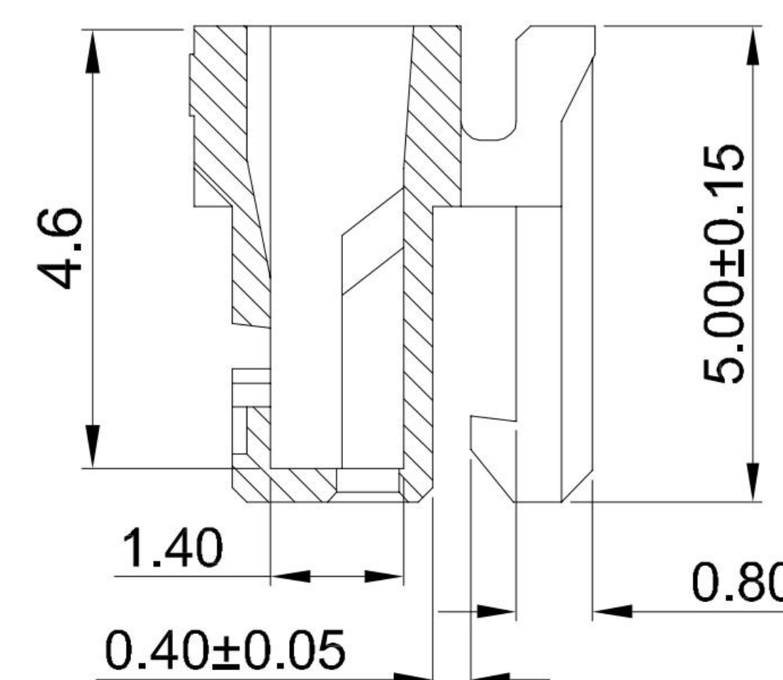
SECTION A-A
