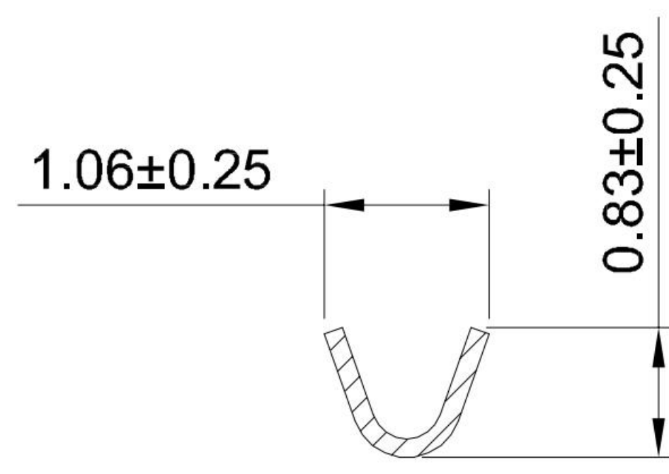
SECION:B-B
