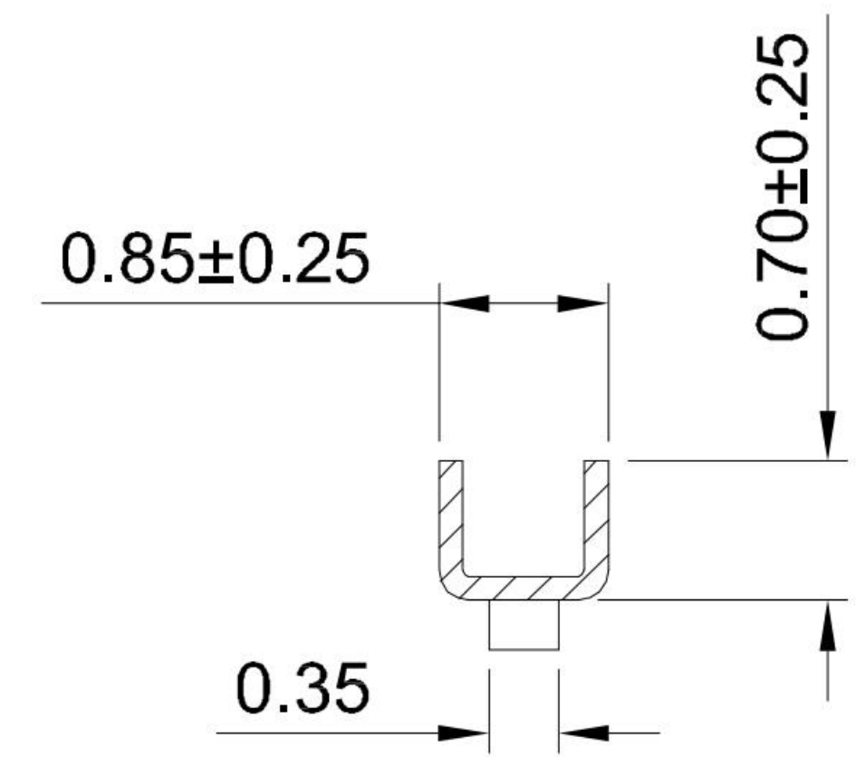
SECION:C-C
