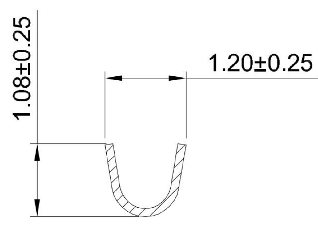
SECION:A-A
