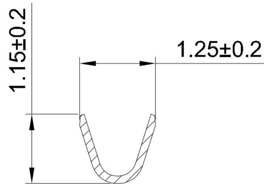
SECTION:B-B
