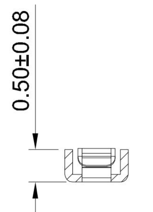
SECTION:D-D
