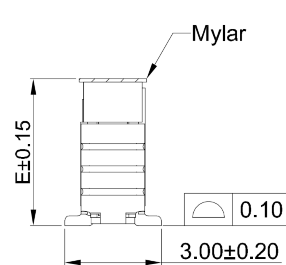
4PIN-5PIN MYLAY
