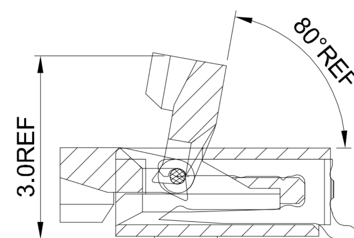
SECCION:A-A
